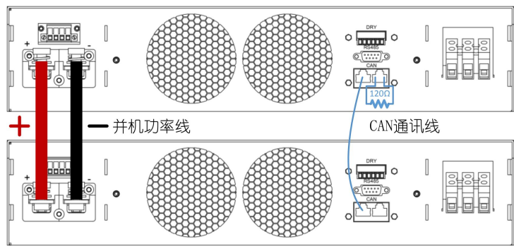
图 4: 并机示意图
