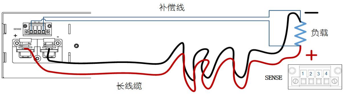
图 3: 电压补偿接线示意图
