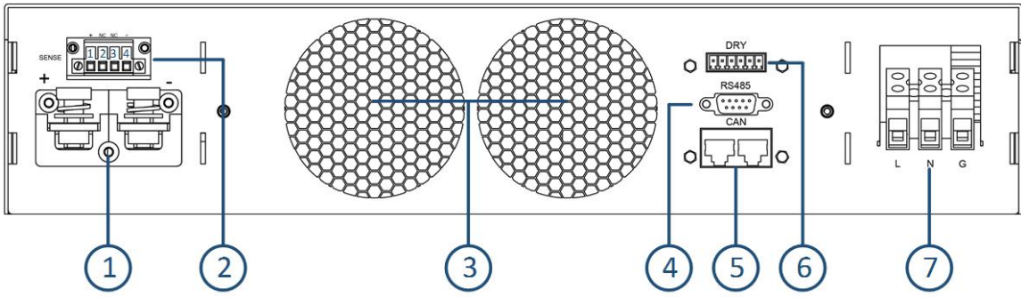
图 1：后面板
