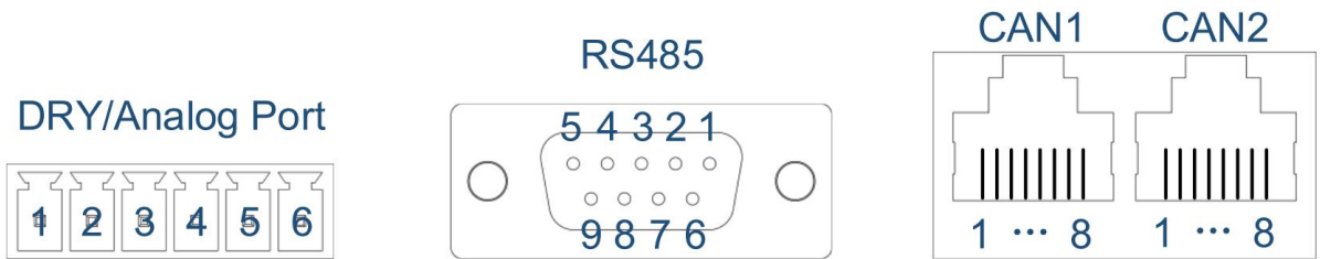
图 2：接口
